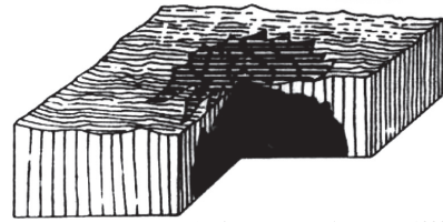
Gambar 3.19 Erupsi Areal
