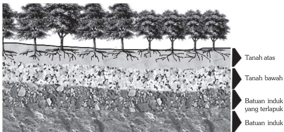
Gambar 3.6 Struktur Tanah
