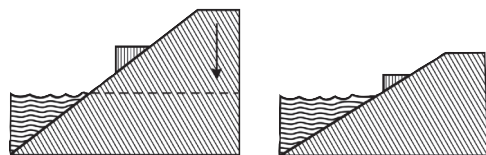
Gambar 3.10 Ilustrasi gerak epirogenetik positif.
