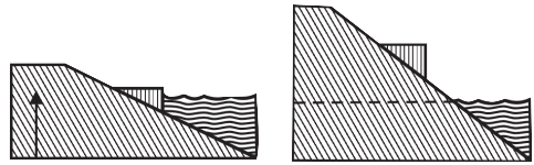
Gambar 3.11 Ilustrasi gerak epirogenetik negatif.
