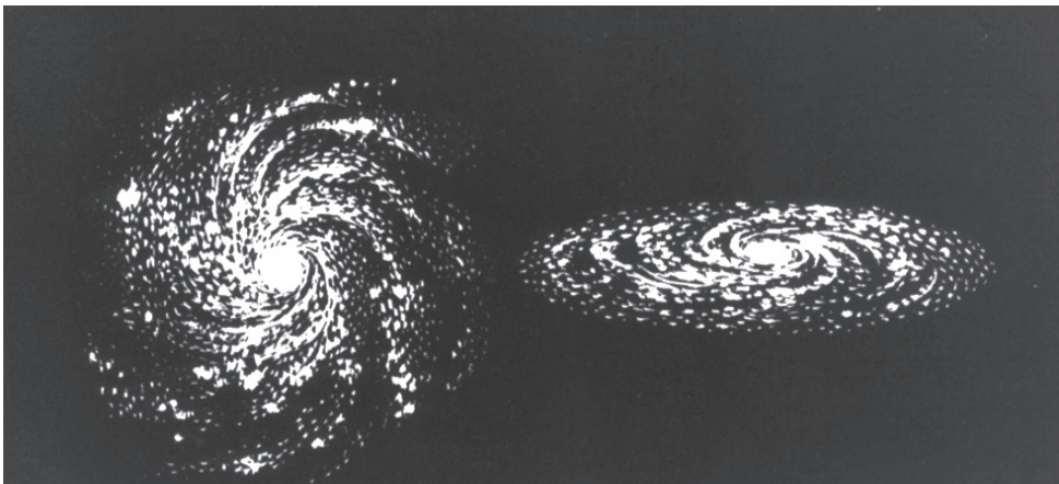
Gambar 2.1 Galaksi
