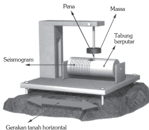
Gambar 3.22 Seismograf Horizontal
