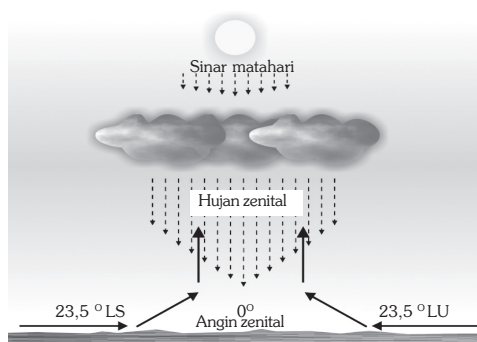
Gambar 4.18 Terjadinya hujan zenital.
