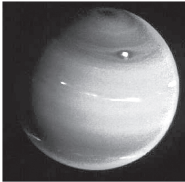
Gambar 2.18 Neptunus yang beku dan dingin.
