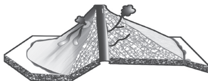
Gambar 3.18 Erupsi campuran
