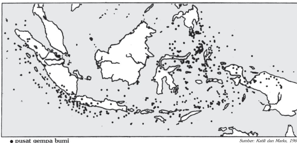
Gambar 3.25 Persebaran gempa bumi di Indonesia.
