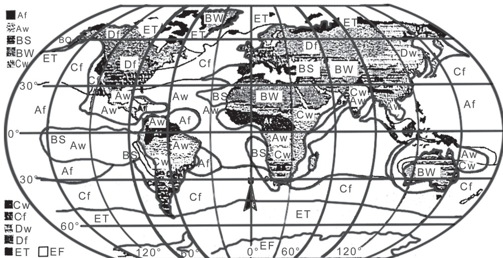
Gambar 4.23 Peta iklim dunia menurut Koppen.
