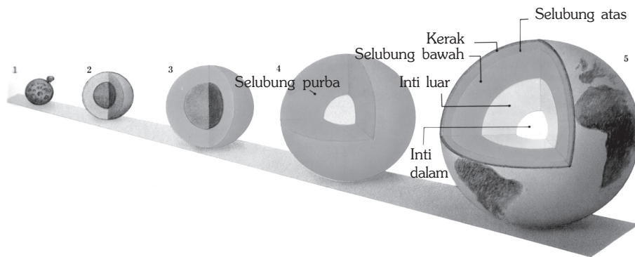
Gambar 2.24 Proses pembentukan lapisan susunan Bumi menurut Rittman.
