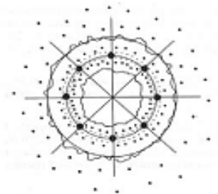
Gambar 7.16 Pola Cincin
