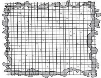
Gambar 7.12 Pola menyebar
