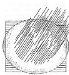
Gambar 7.14 Pola Memusat
