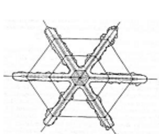
Gambar 7.15 Pola Bintang
