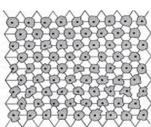
Gambar 7.13 Pola Galaktika
